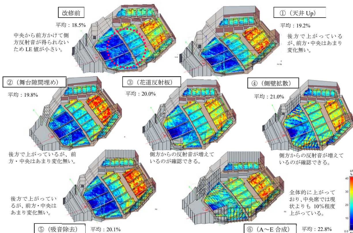
図3 改修方法の比較 (LE 値)
