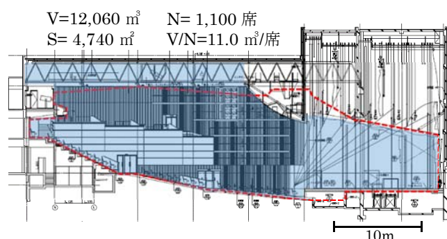
図2 断面図(赤破線：改修前)
