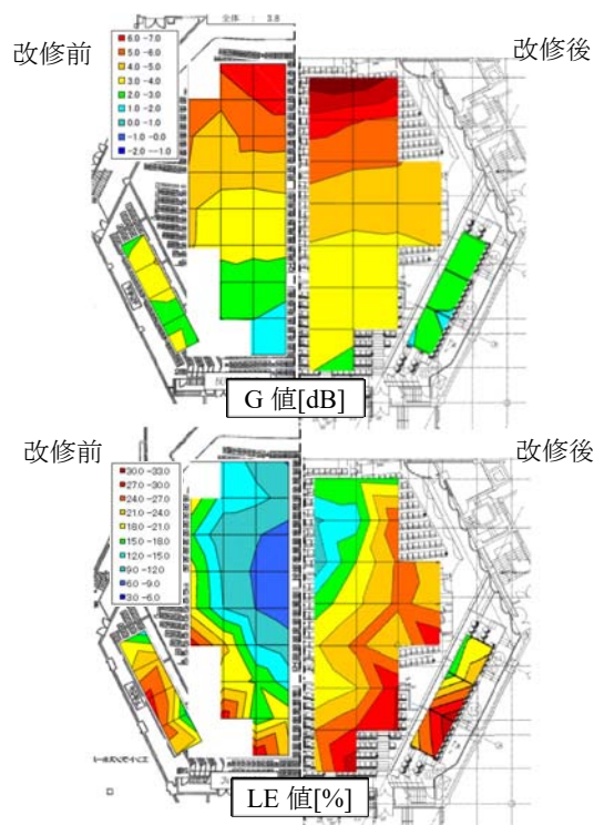
図6 G 値、LE 値測定結果 改修前後比較
